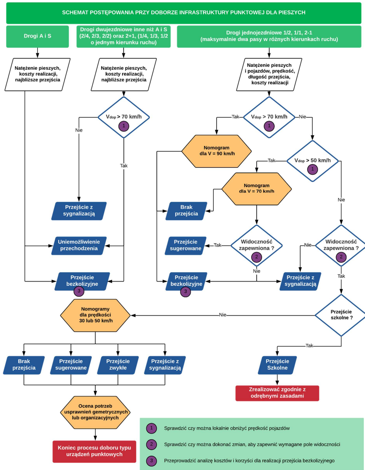
Rys. 8.4.1. Schemat postępowania przy doborze rodzaju infrastruktury punktowej dla pieszych na drogach zamieszkanych i ulicach
